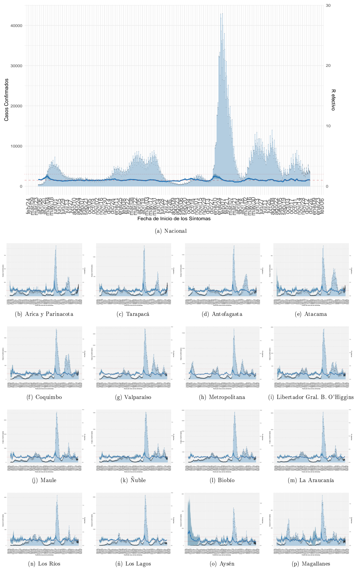
Figura 5: Casos de COVID-19 confirmados y estimados; Número efectivo reproductivo diario, calculado sobre la base de los últimos 7 días, al 25-12-2022 .
