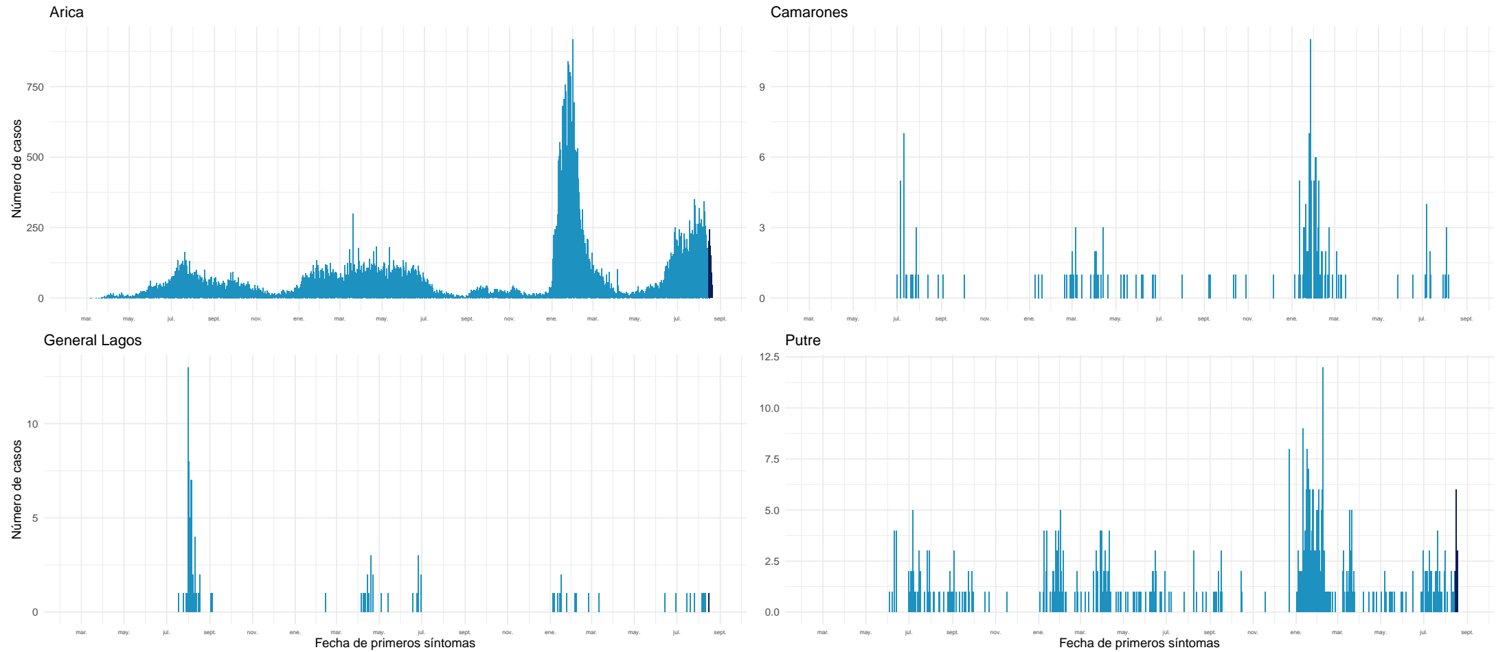
Figura 19: Curva epidémica de casos COVID-19 según comuna de residencia, región de Arica y Parinacota, al 21-08-2022 (casos activos en azul oscuro).
