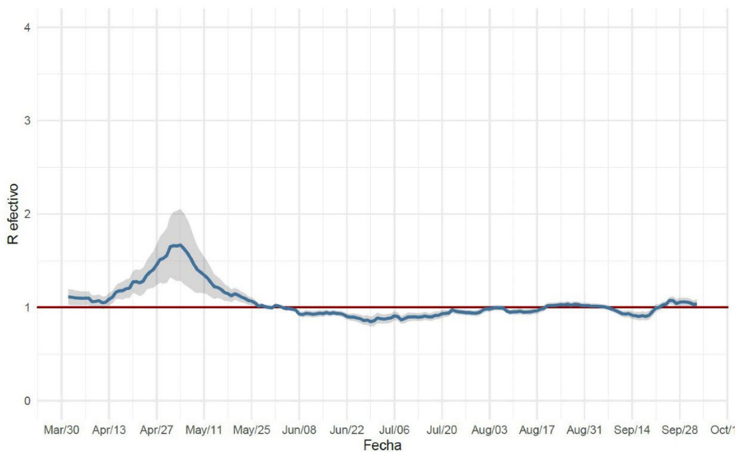
Figura 5. Número efectivo reproductivo diario a nivel nacional y regional, calculado sobre la base de los últimos 7 días. Chile, al 04 de octubre de 2020.
