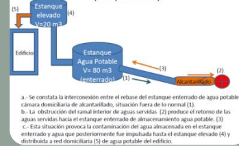
Sistema Agua Potable-servida de edificio (simplificado)
